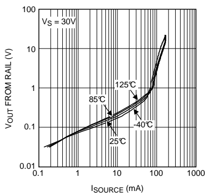
输出摆幅与拉电流间的关系
